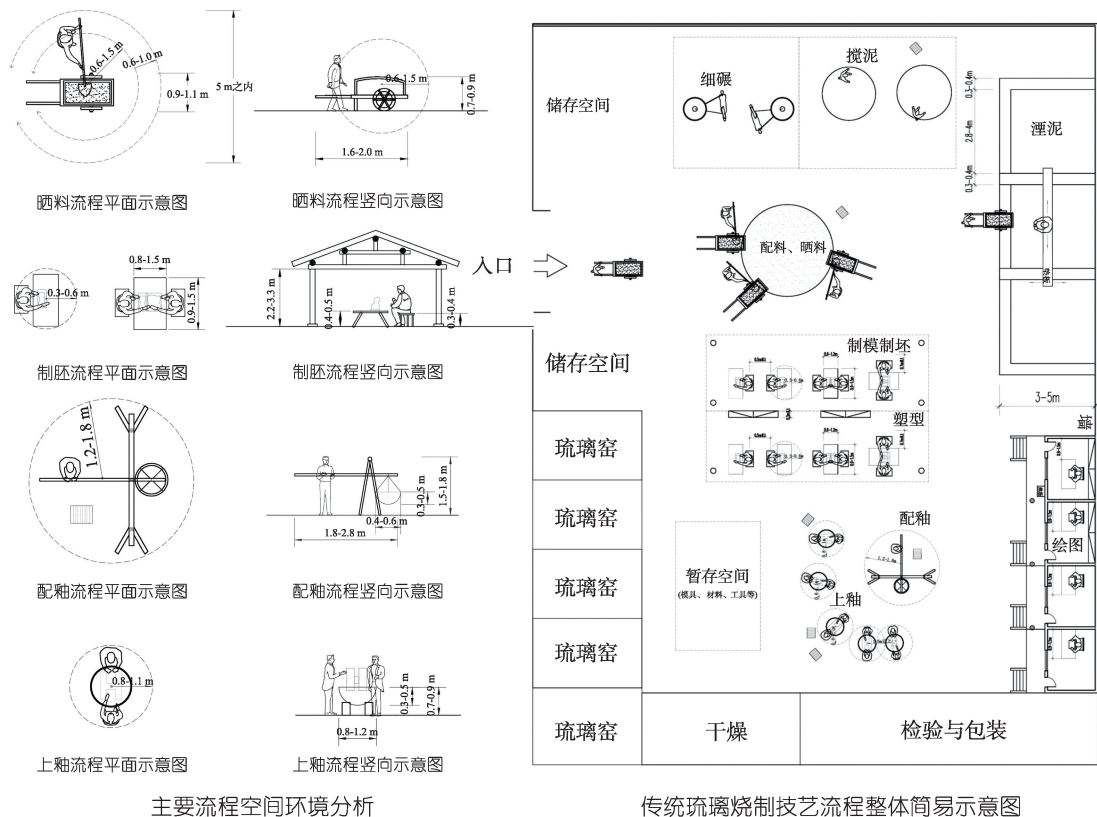
图8 琉璃烧制技艺空间环境分析
